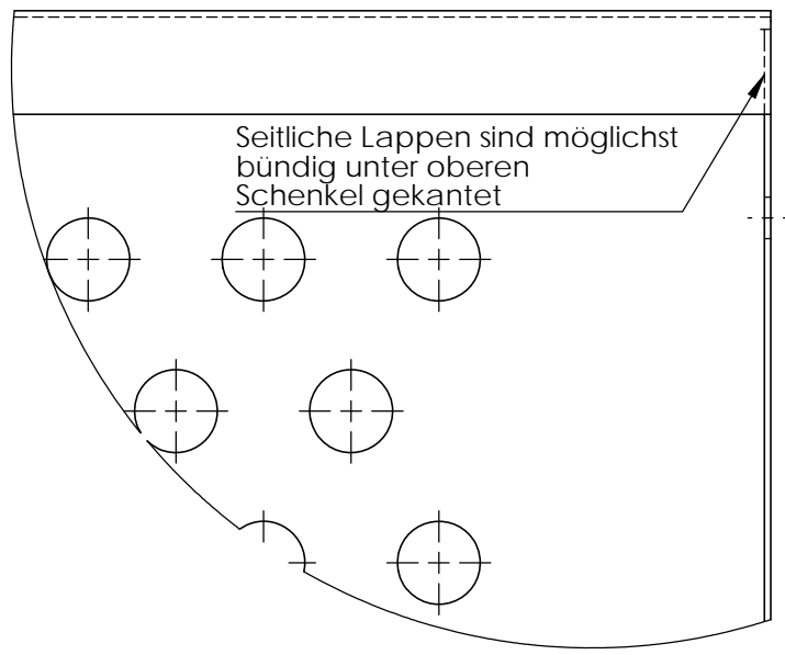
Ansicht innen Schnitt A-A
